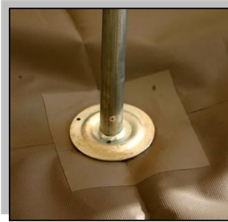
Fußplatte bei beiden Mittelstäben!
