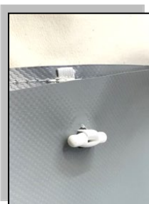
Mittelstangen in Rahmenkonstruktion ohne Ösen im Firstbereich!
